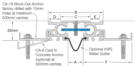
CA-25 - CA-50
